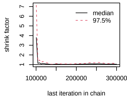
d.Erlotinib.Erlotinib_MMPi
