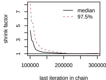
d.Erlotinib.Erlotinib_Autophagy
