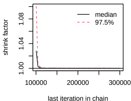
d.Afatinib.Placebo
