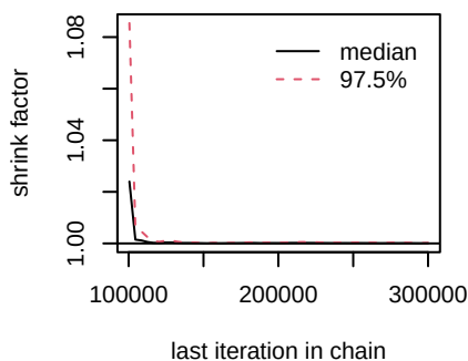
d.Erlotinib.antiangio
