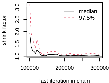
d.Erlotinib.Erlotinib_ERi
