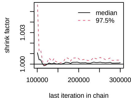
d.Gefitinib.Gefitinib_antiangio
