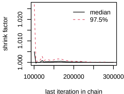
d.Erlotinib.Erlotinib_antiangio
