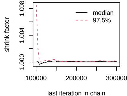
d.Osimertinib.Osimertinib_chemo
