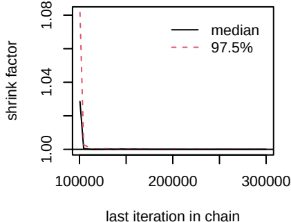
d.Gefitinib.Lazertinib
