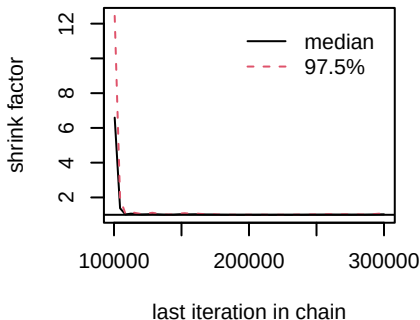
d.Erlotinib.Rociletinib
