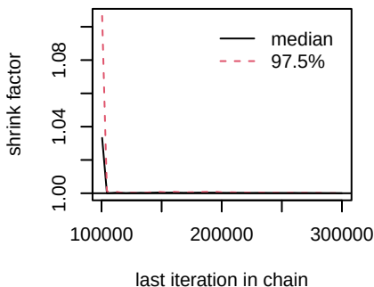
d.Gefitinib.Gefitinib_chemo
