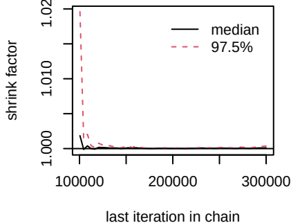
d.Osimertinib.Osimertinib_antiang
