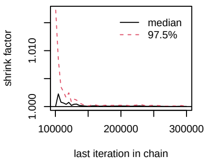
d.chemo.Osimertinib
