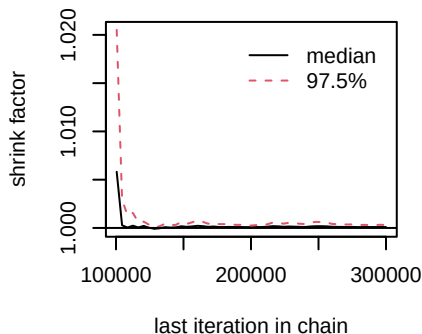
d.Erlotinib.Erlotinib_HER3i
