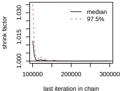
d.Erlotinib.DHFRi
