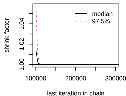
d.Erlotinib.Dacomitinib
