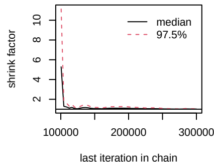
d.Erlotinib.Erlotinib_HGFi
